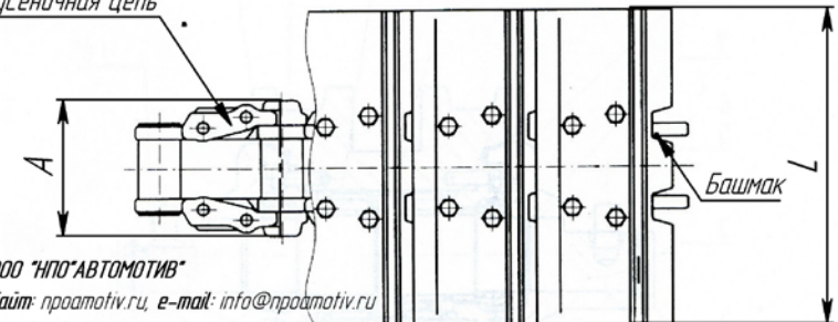
Гусеничная цепь
