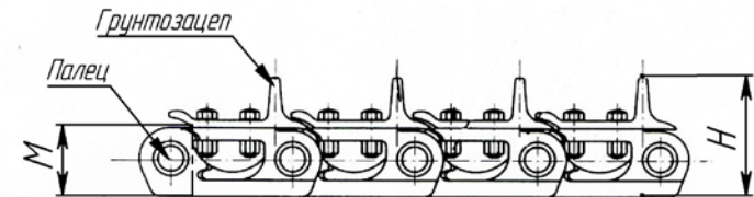
Чертеж гусеничной цепи в сборе с башмаком
