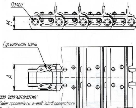
Чертеж гусеничной цепи в сборе
