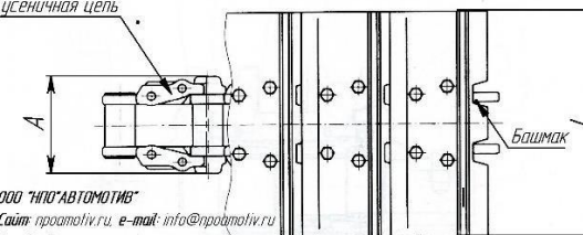
Гусеничная цепь
